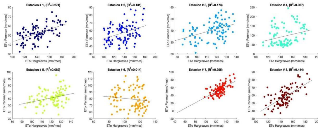
Figura 4. Relaciones entre ETO usando ecuaciones de Penman-Monteith y Hargreaves-Samani para valores mensuales.
