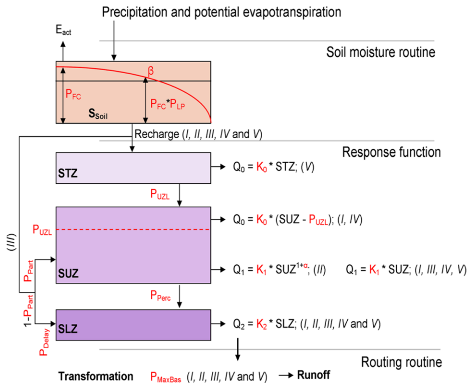
Figura 1. Esquema de funcionamiento del modelo HBV.
