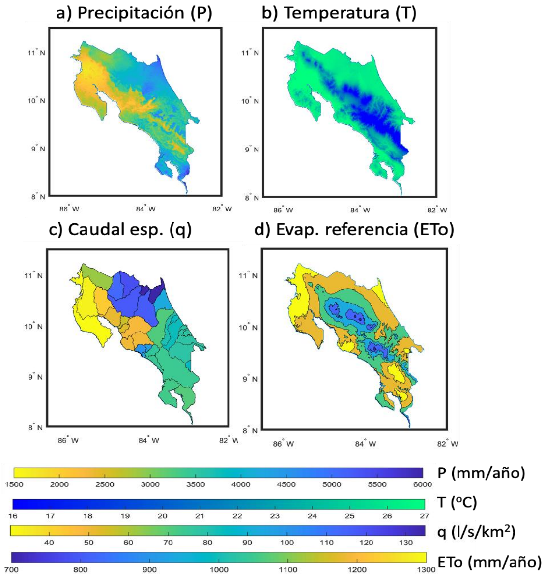
Figura 2. Promedios anuales (1990-2020) de diferentes variables que provienen de las observaciones y que fueron usadas en el balance de aguas.
